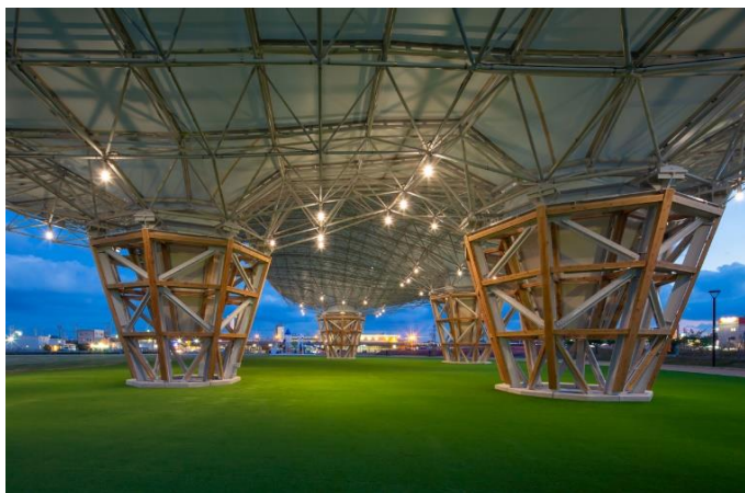
内観（立体トラス）
